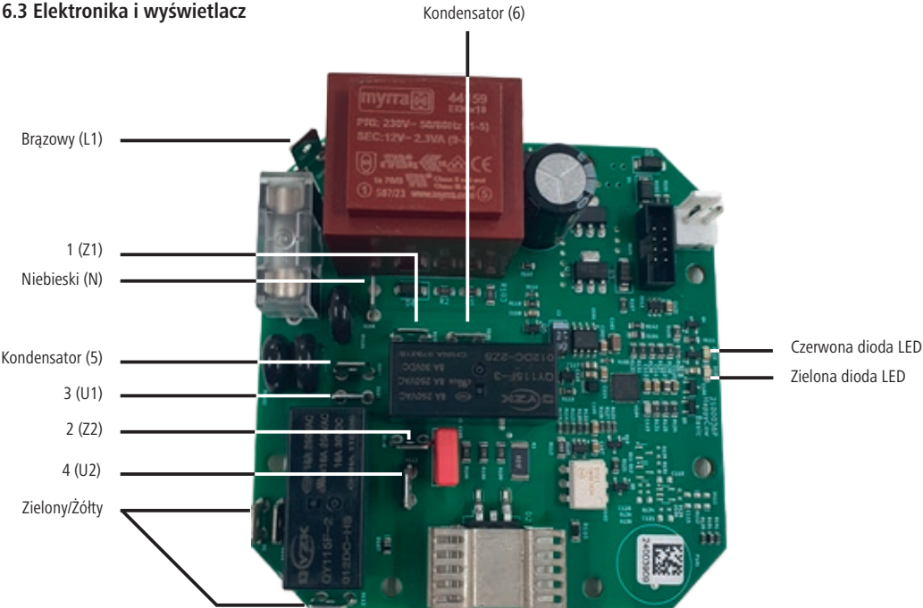
Rysunek 5: Schemat podłączenia płyty z kondensatorem – MaxiSwing
