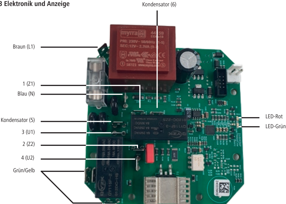
Abbildung 5: Anschlussschema der Platine mit Kondensator
