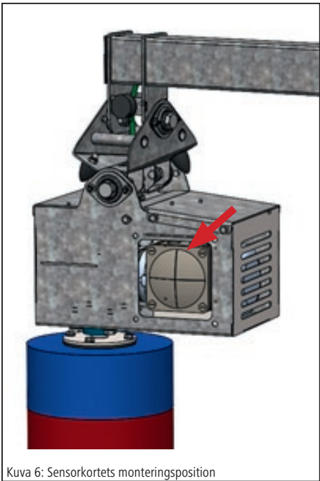
Kuva 6: Sensorkortets monteringsposition
