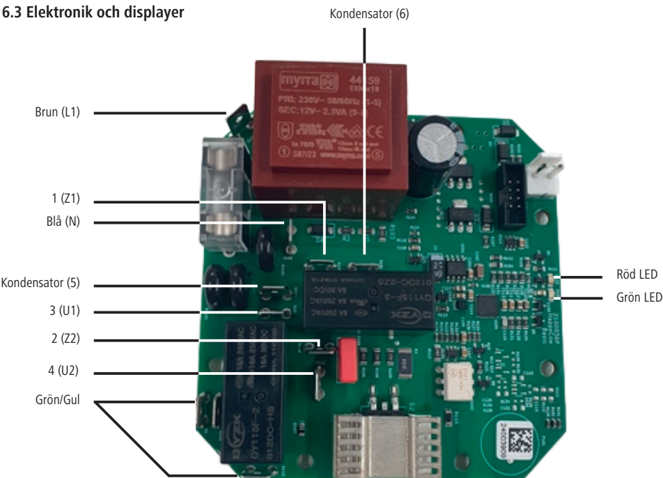
Bild 5: Kopplingsschema för kretskortet med kondensator - MaxiSwing
