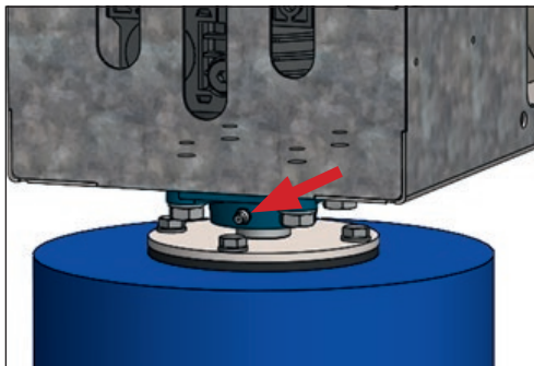
Abbildung 7 – Position Schmiernippel
