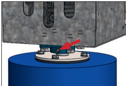
Figure 7 – Position des graisseurs
