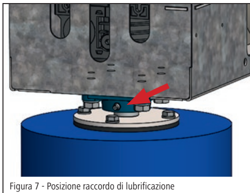
Figura 7 - Posizione raccordo di lubrificazione
